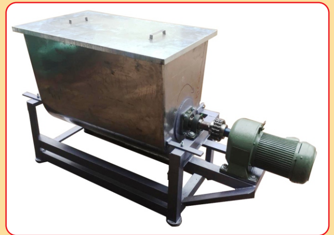
DRY MATERIAL 20KG, 30KG, 60KG KIỂU DÁNG MÁY TRỘN 20KG, 30KG, 60KG
